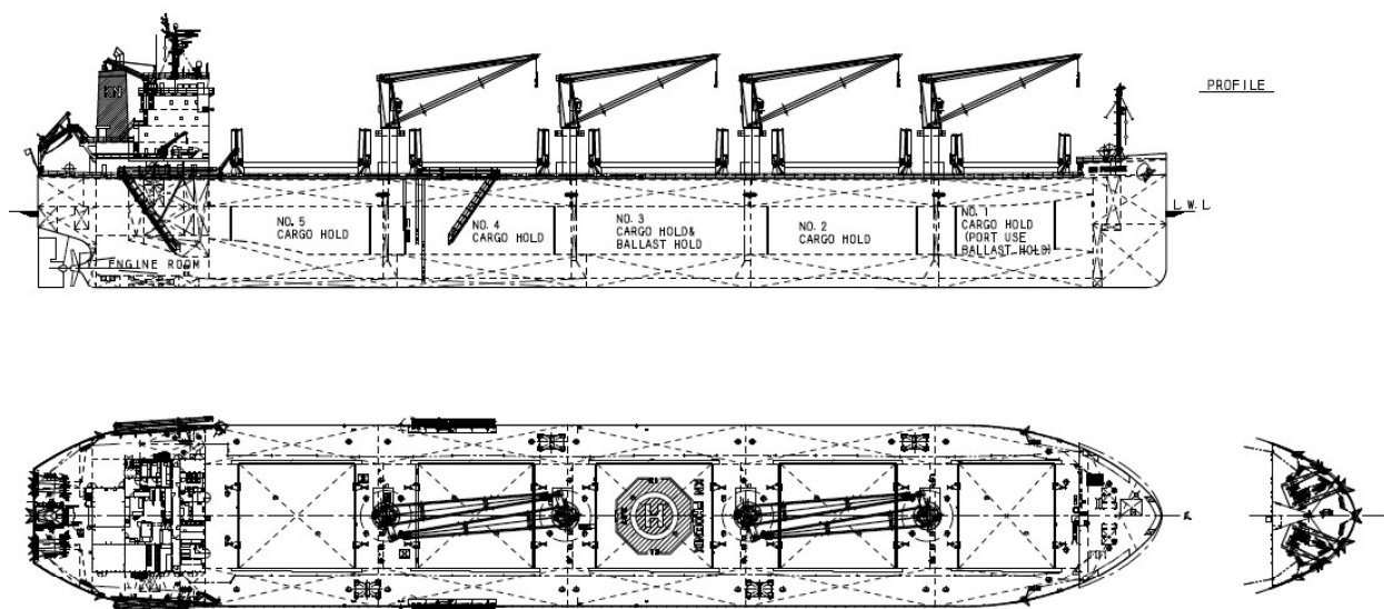
一般配置図
