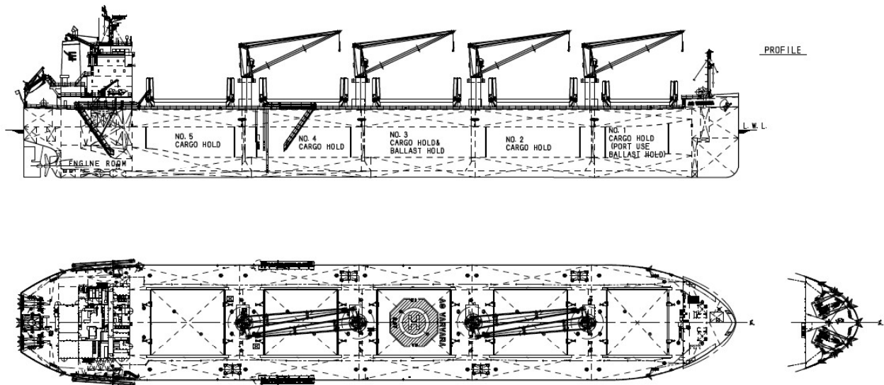
一般配置図
