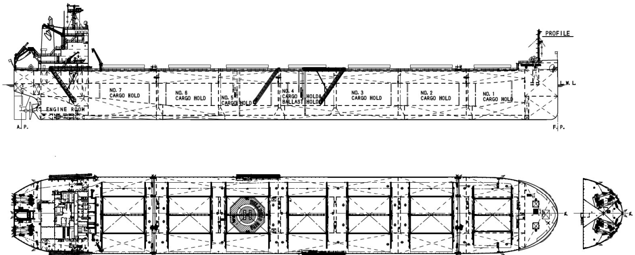
一般配置図
