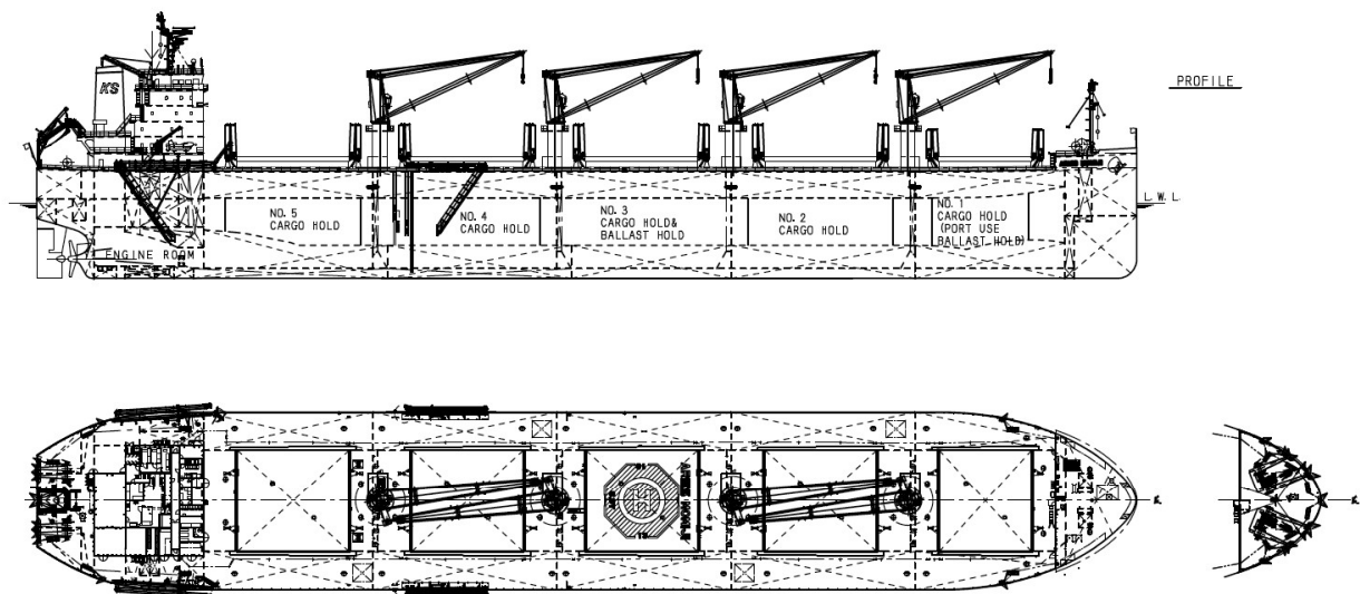
一般配置図
