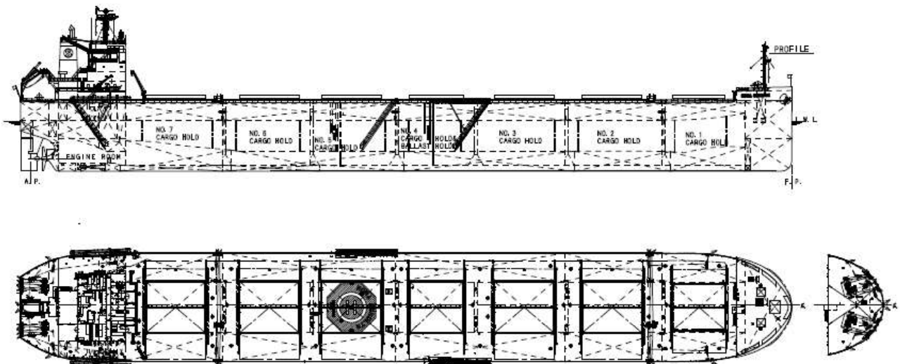
一般配置図
