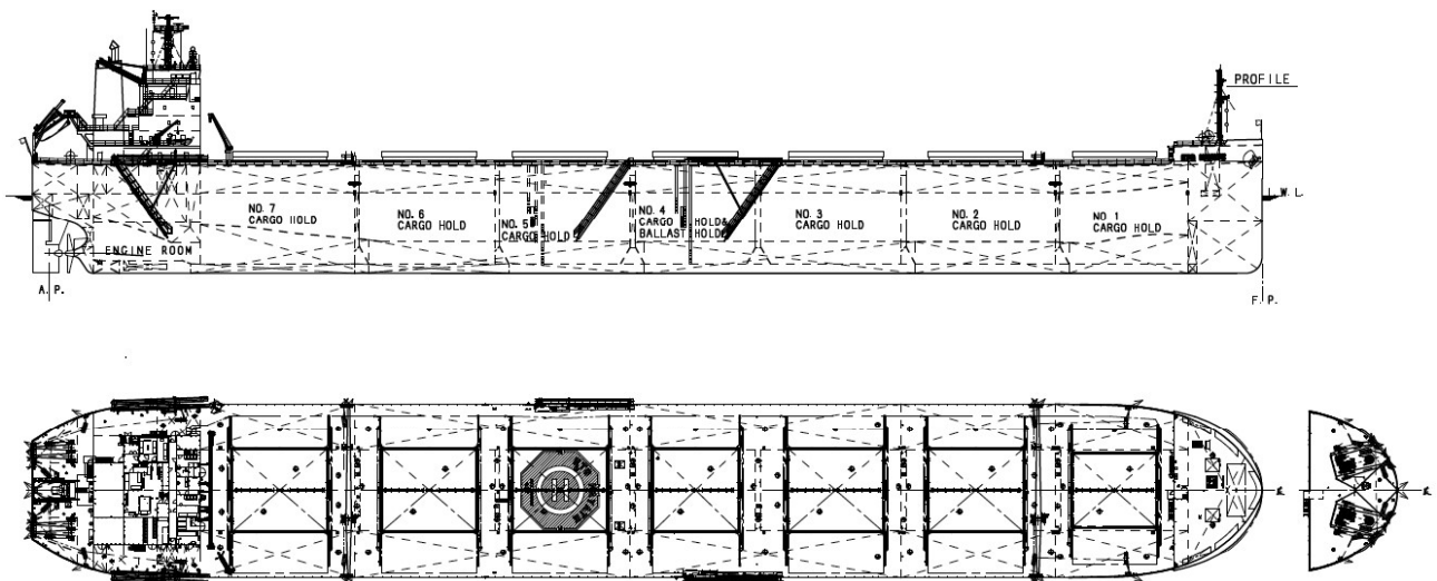
一般配置図
