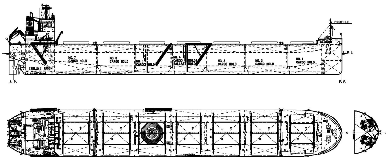
一般配置図
