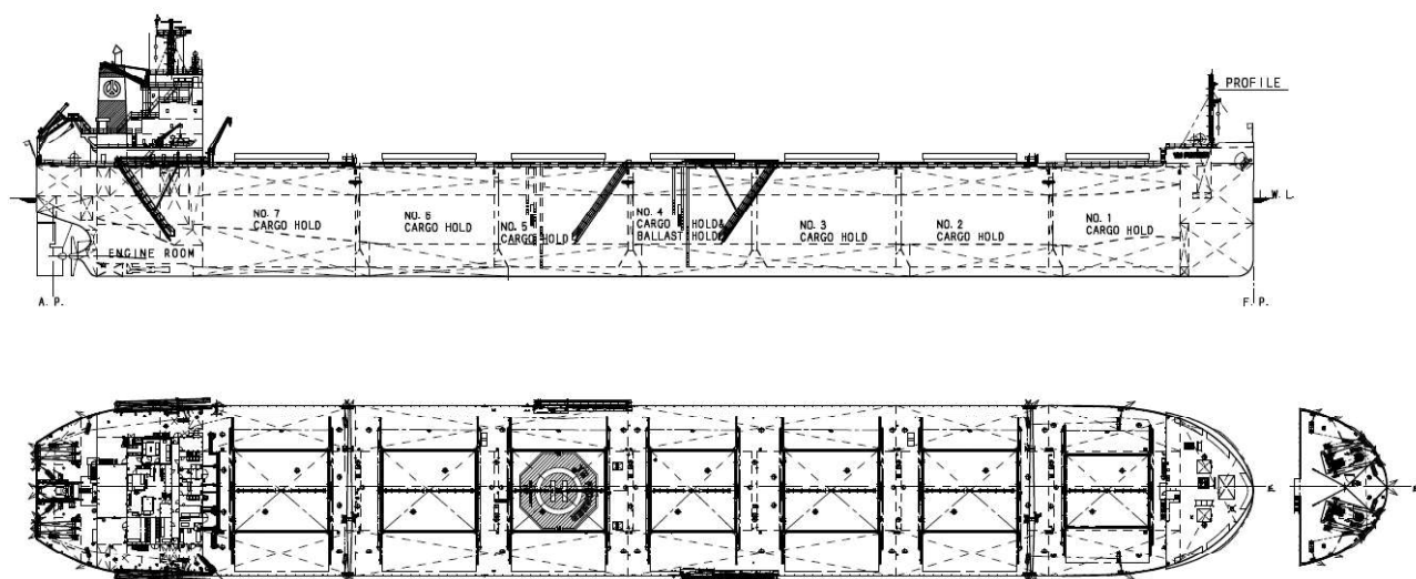
一般配置図
